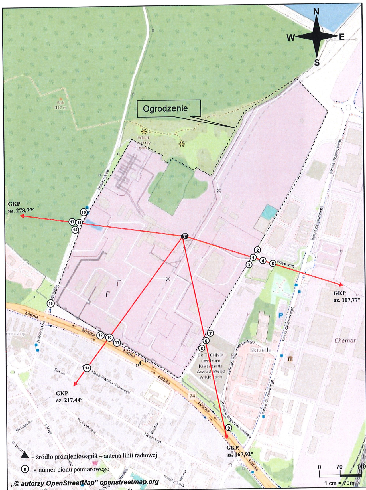
Rys. 1. Usytuowanie punktów i pionów pomiarowych w otoczeniu instalacji radiokomunikacyjnej Stacja Netia KIELW001-KIELM00045 Kielce, ul. Hubalczyków 30
